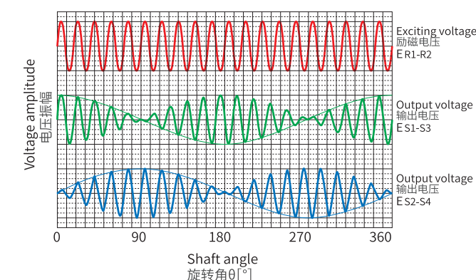
图2 励磁·输出电压特性(+方向旋转)
