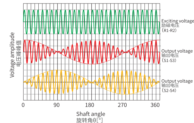
图4 1X的输出电压变化
