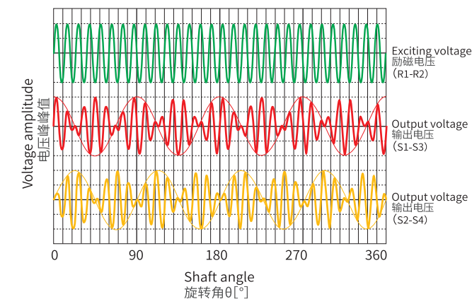
图5 4X的输出电压变化
