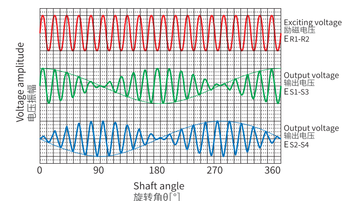
图3 励磁·输出电压特性(-方向旋转)
